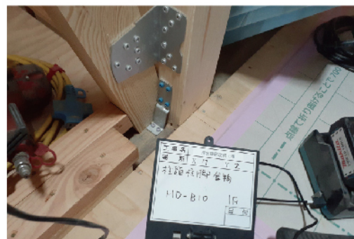
柱頭柱脚金物で補強
