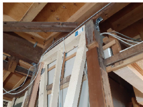
耐力壁の金物取付
